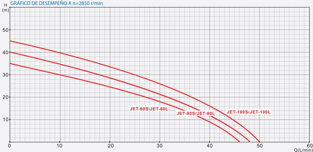
GRÁFICO DE DESEMPEÑO A n=2850 r/min
